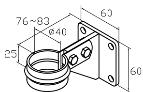
リングフック52
