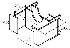
トルクレンチフック QLE1000N2(東日)用
