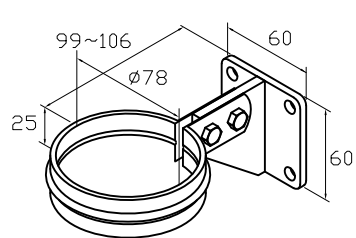
リングフック76
